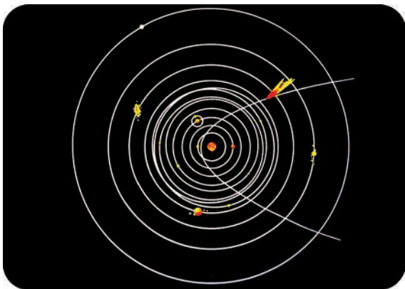
ՄԵՐ ԱՐԵԳԱԿԼԱՅԻՆ ՀԱՄԱԿԱՐԳԸ
